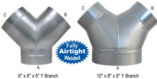
6" x 6" x 6" Y Branch
